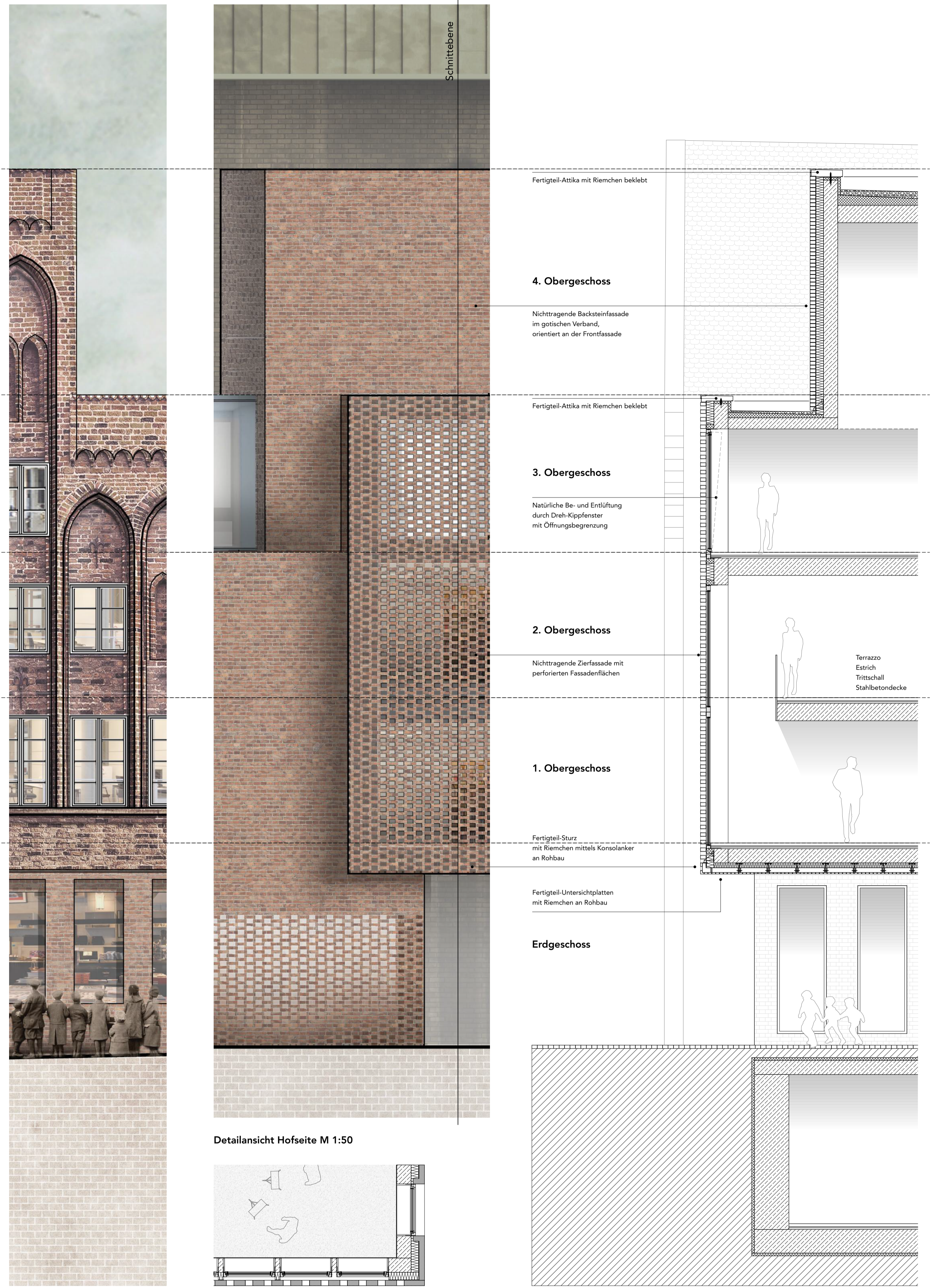
Detailansicht Straßenseite M 1:50
