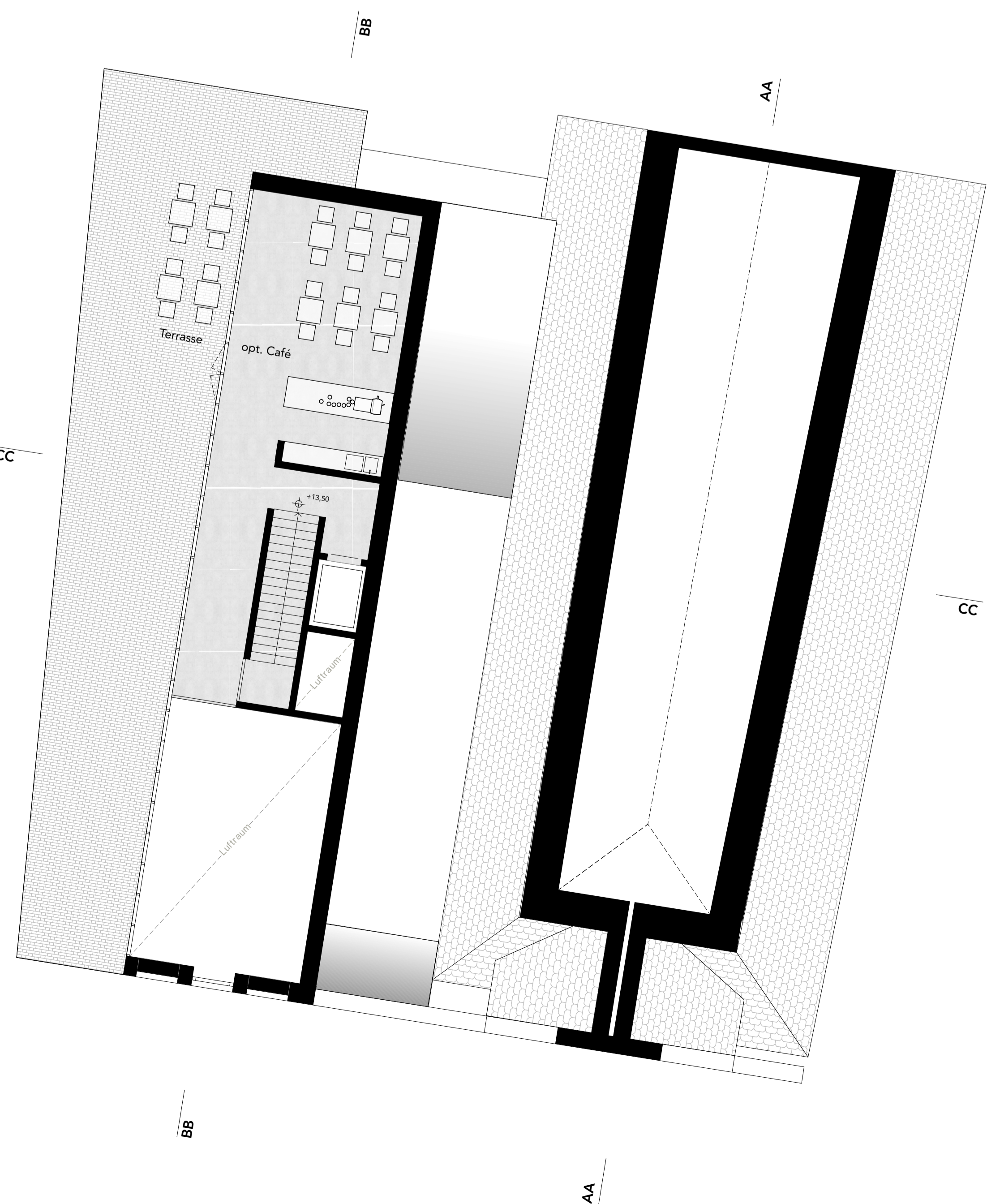
Grundriss 4.OG M 1:100
