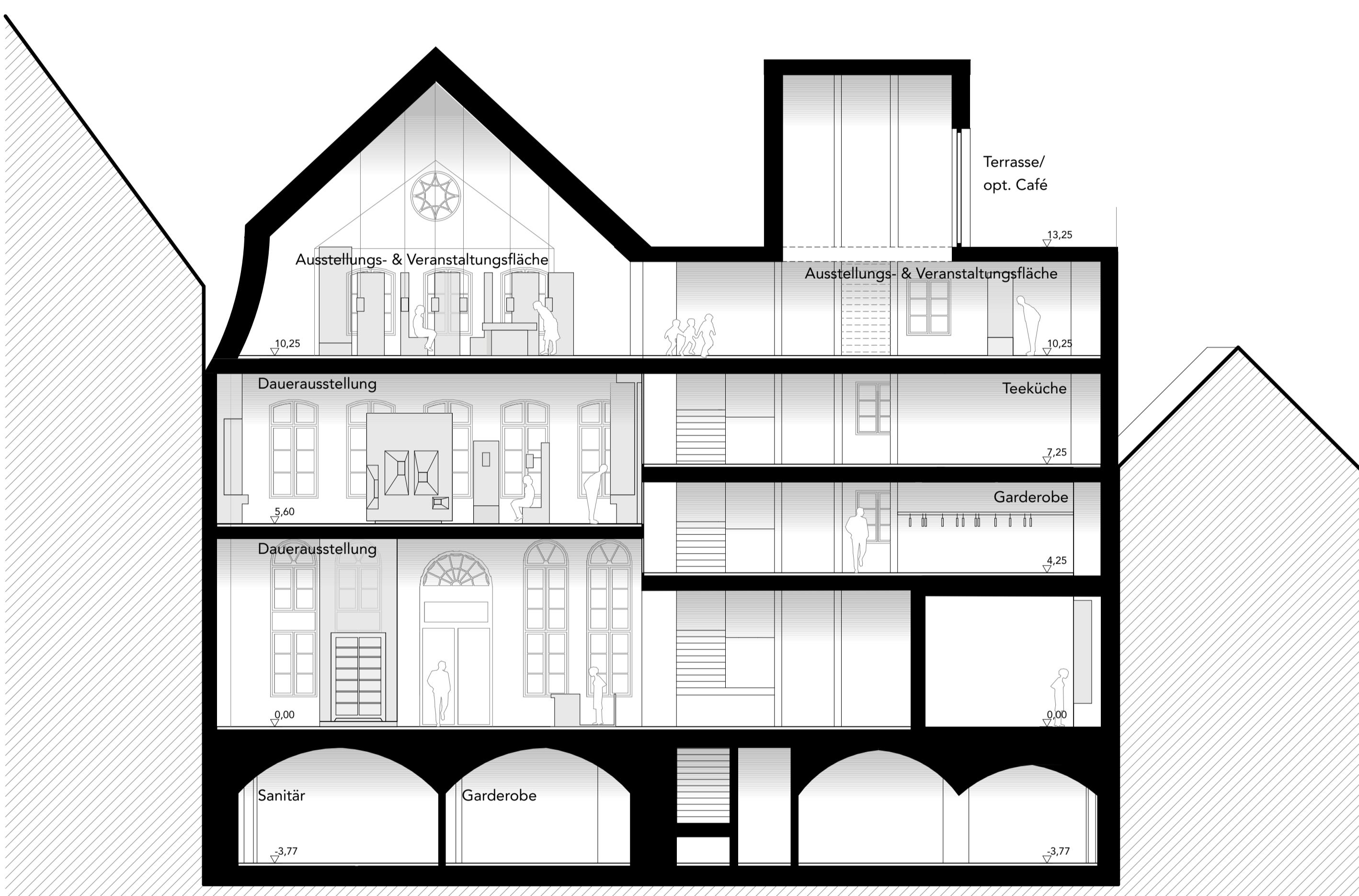
Querschnitt CC M 1:100
