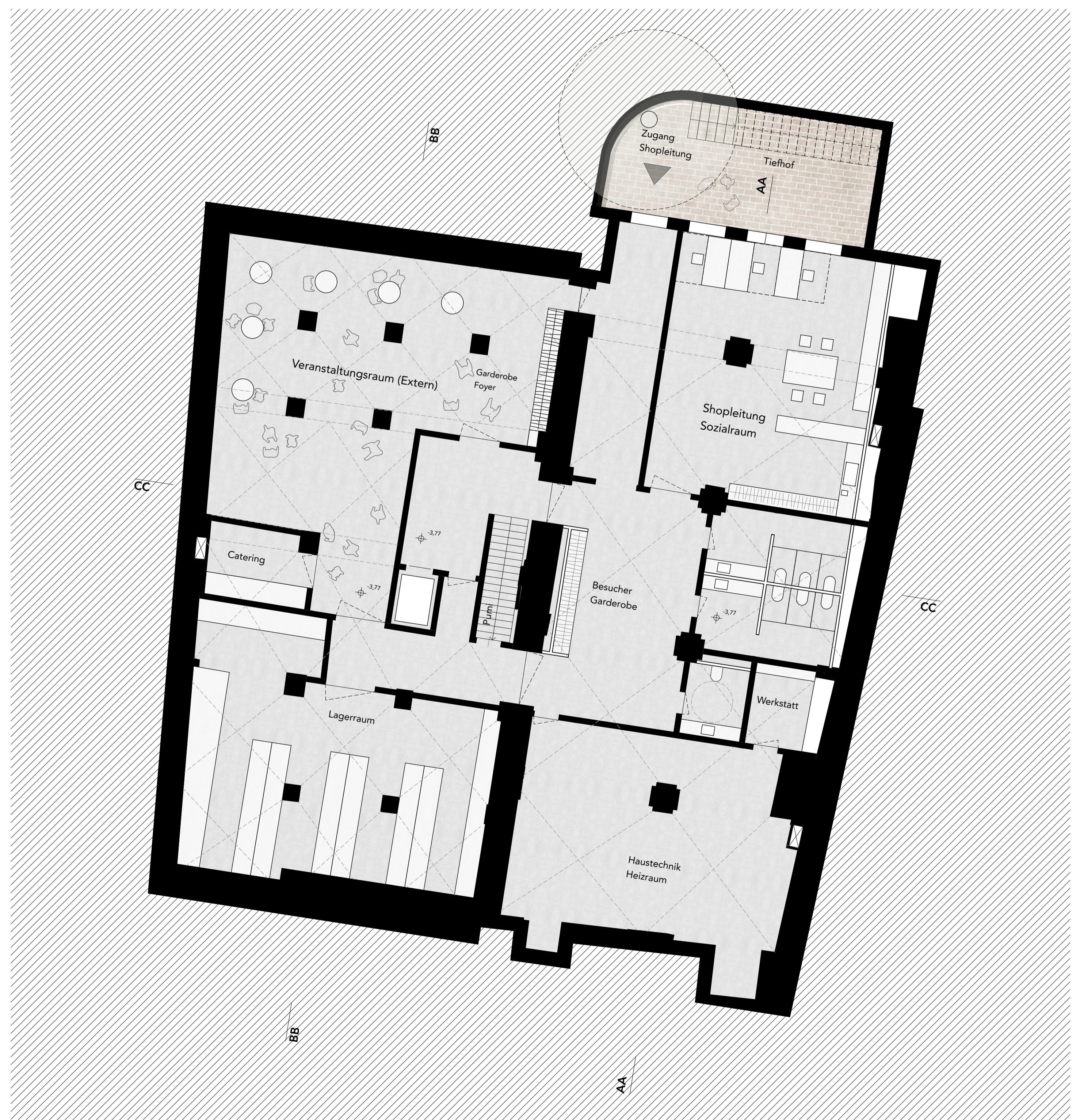
Grundriss UG M 1:100
